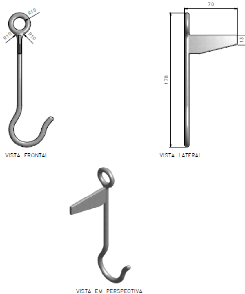
Figura 1 - Gancho para isolador roldana
